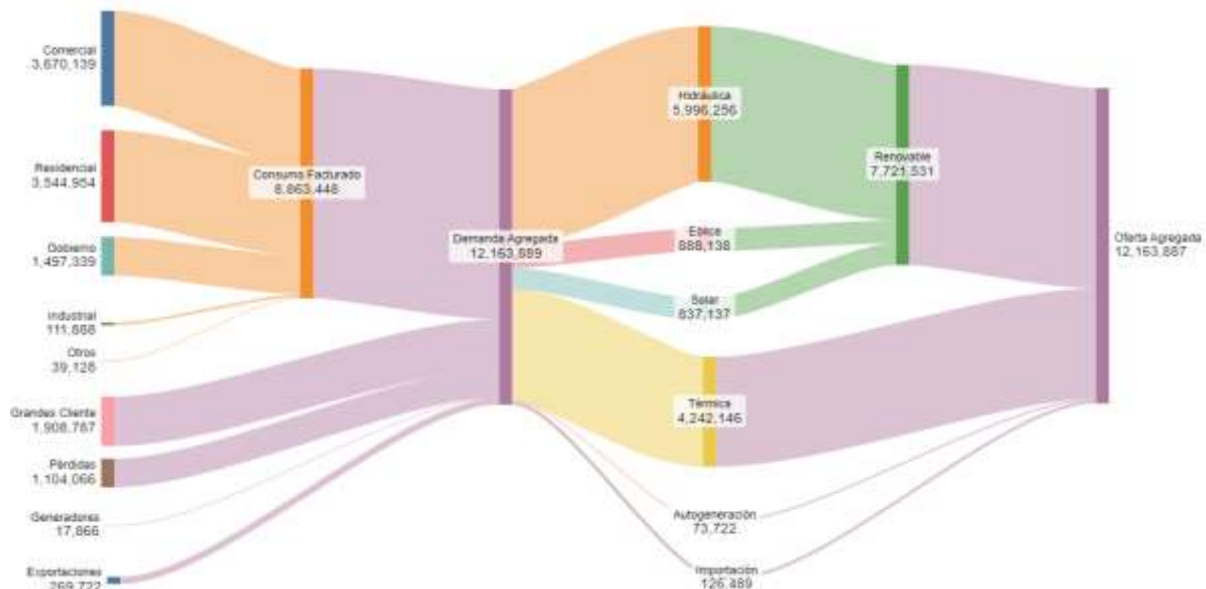
Gráfica No.1-5 OFERTA Y DEMANDA AGREGADA DE ELECTRICIDAD ENERO-DICIEMBRE DE 2023 (En miles de Kwh)
